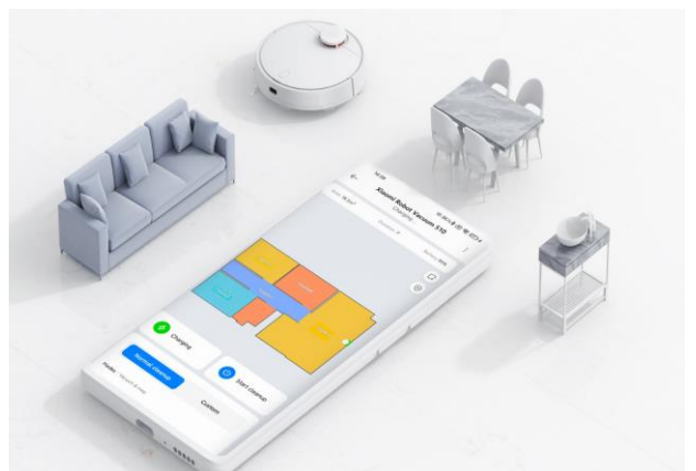
Funkcije mapiranja
